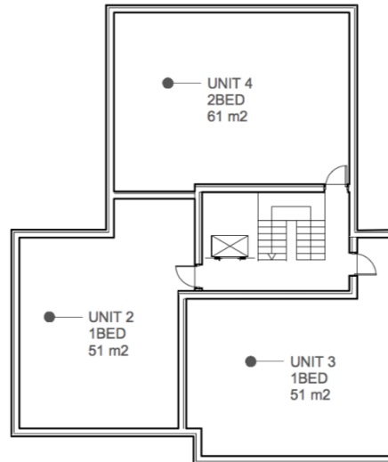
2 FIRST FLOOR Scale: 1:200
